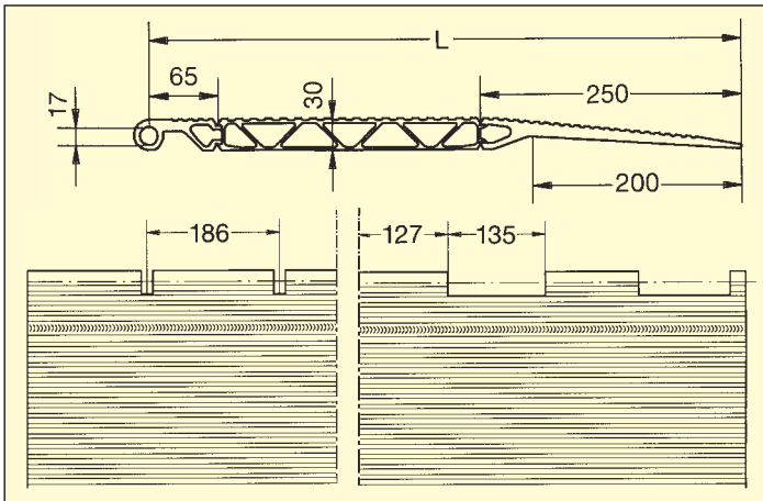
Versio 3:n liitäntärakenne
